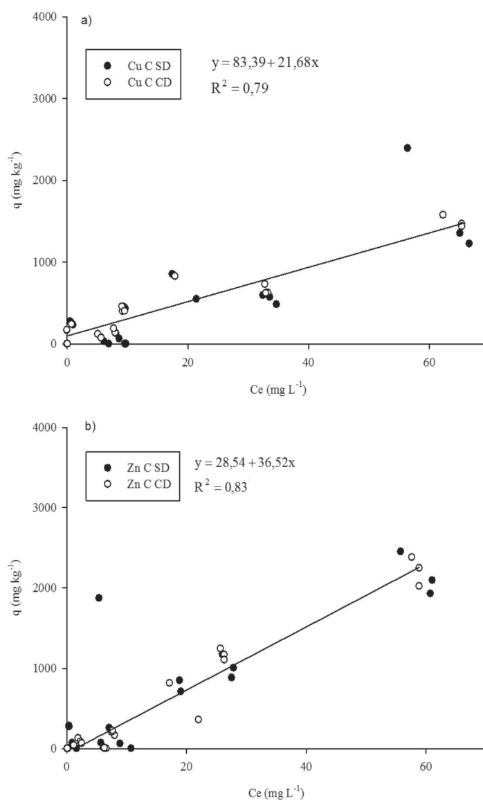
Figura 2. Isotermas de adsorção de Cu e Zn competindo a pH 5,5 e força iônica 15 mmol L -1 em Latossolo. a) Adsorção de Cu competindo no tratamento sem dejetos suínos (SD) e com dejetos (CD); b) Adsorção de Zn competindo no tratamento sem dejetos suínos (SD) e com dejetos (CD).
